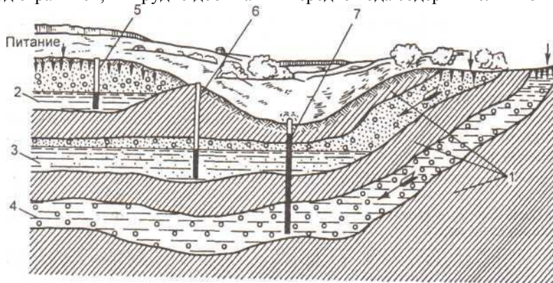
Рис. 1.4.2.1 - Схема залегания подземных
